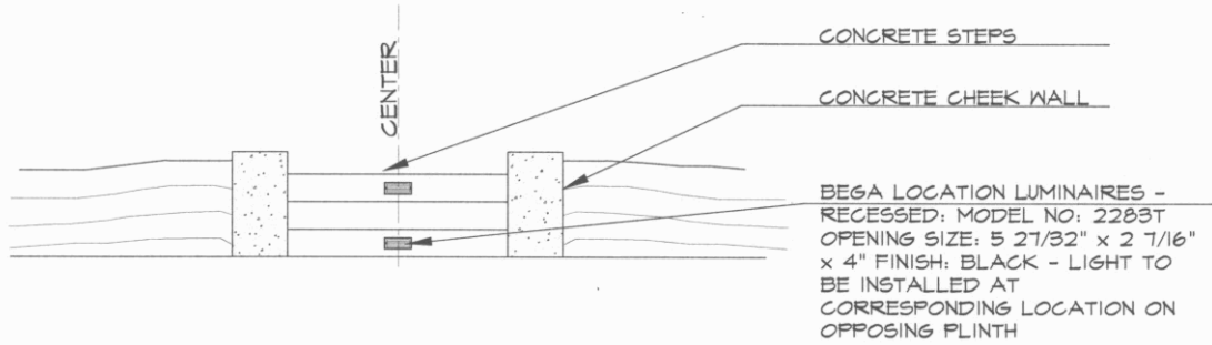
ELEVATION
